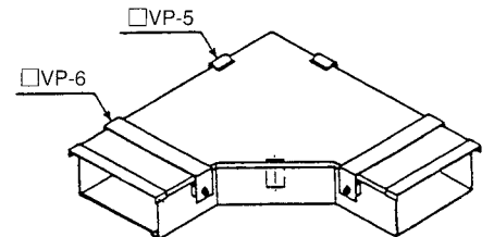
平カブセ蓋 L型
