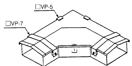
山型カブセ蓋 L型
